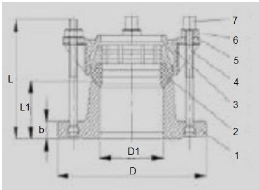
Рис.2. Муфта ПФРК.
